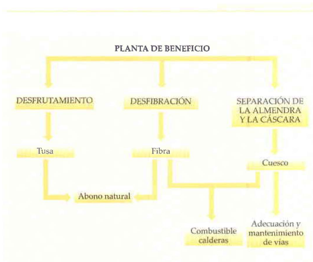
Figura 5. Diagrama de flujo de los subproductos sólidos
