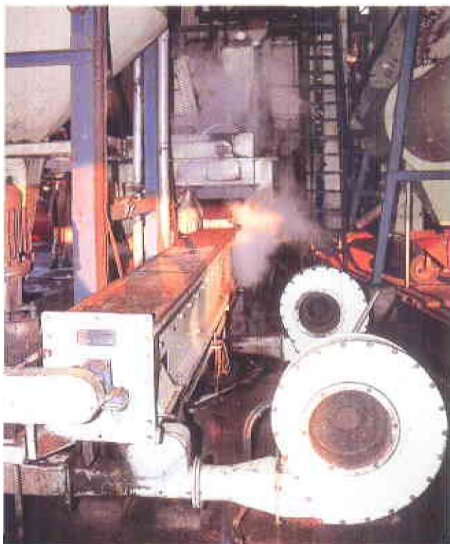
Equipos integrados en la sección de palmistería
